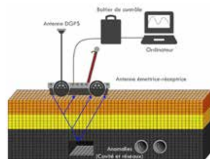
Principe de fonctionnement du geo radar
